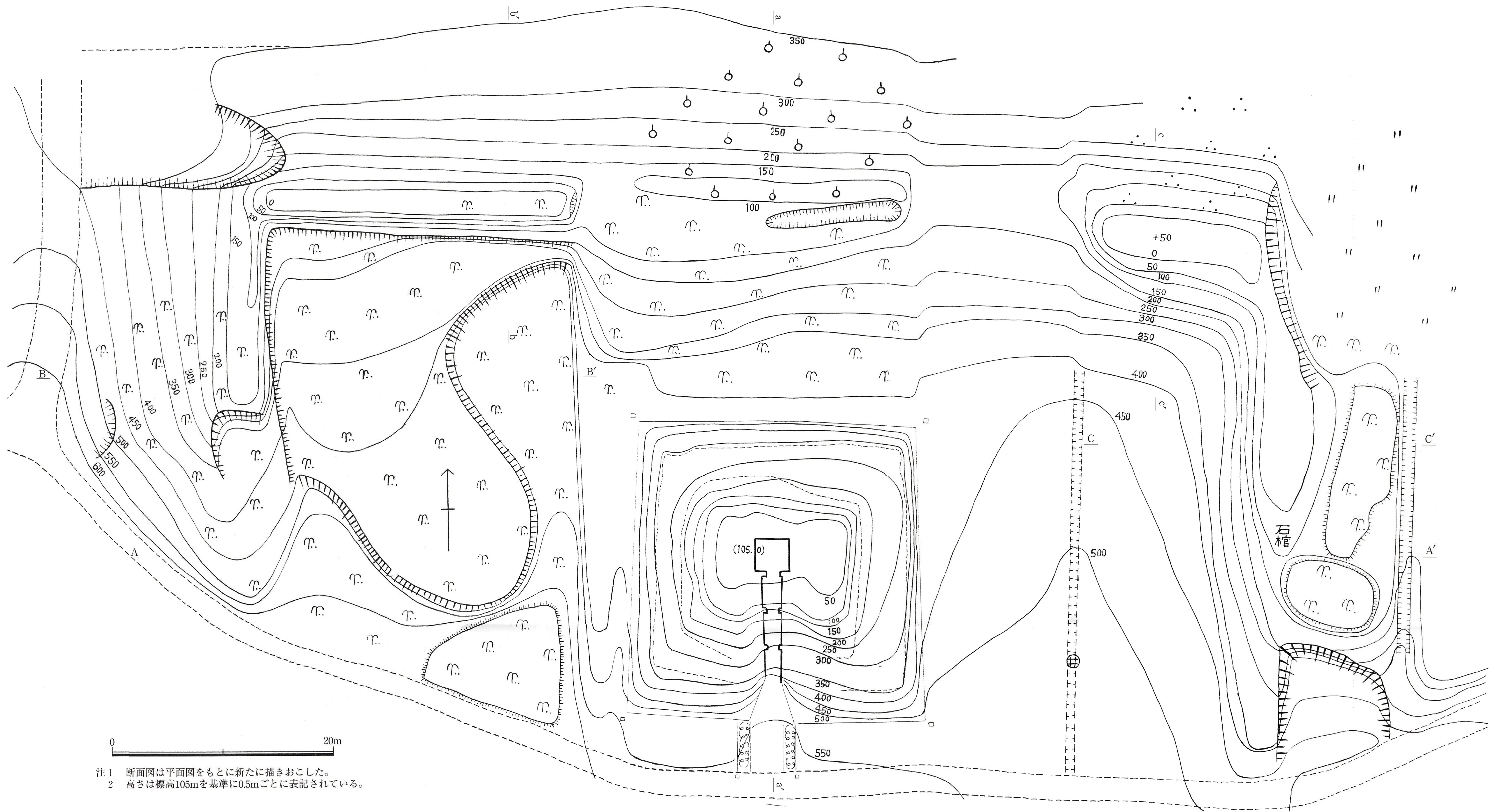
付図1 黄金塚陵墓参考地 墳丘及び外堤平面図・断面図 [昭和33年作成] (1/200)
