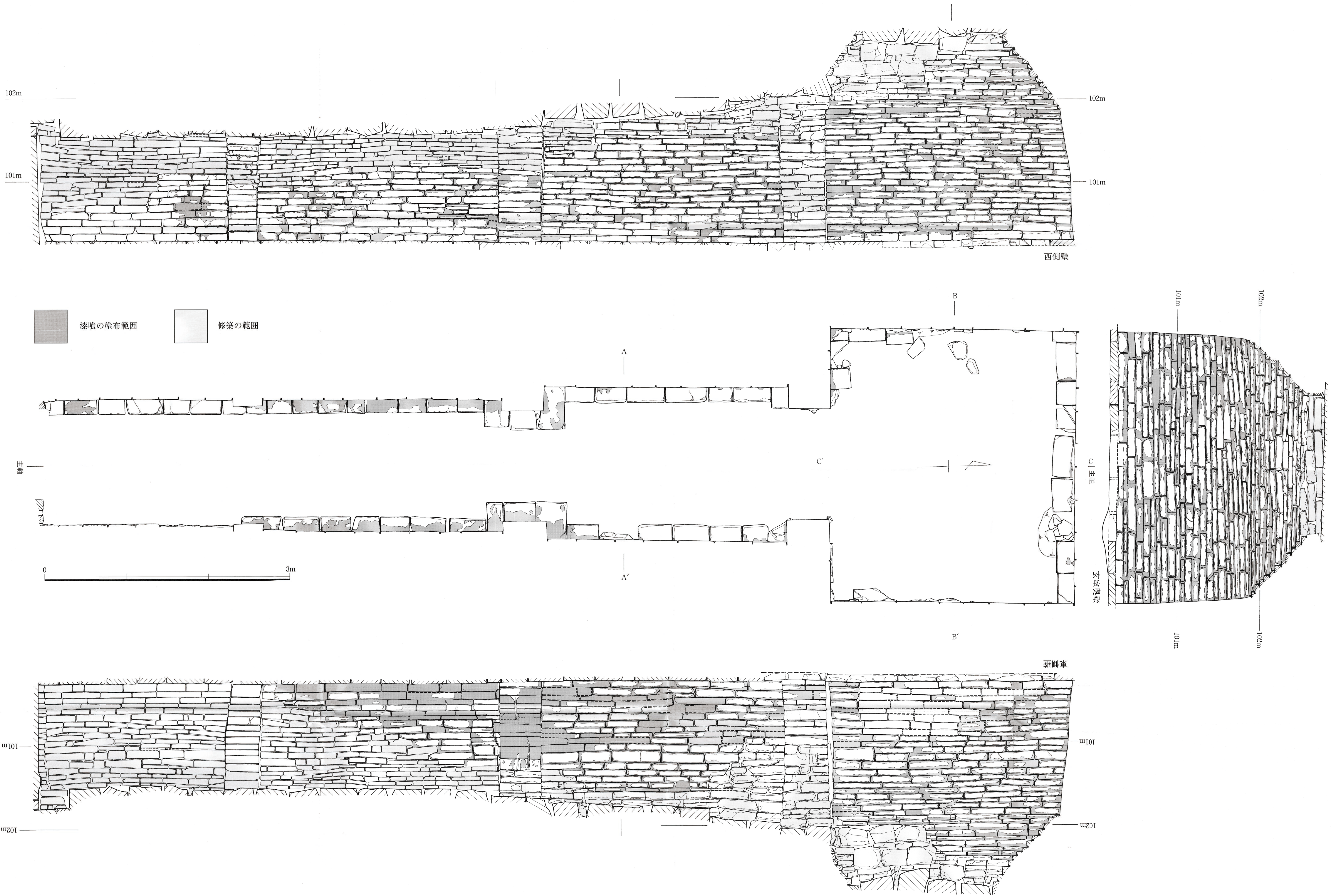
付図2 黄金塚陵墓参考地 石室実測図(1) (1/20)
