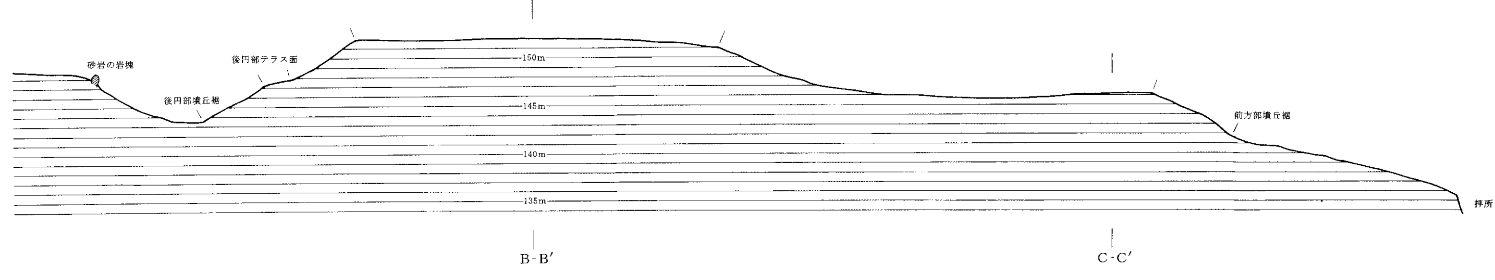
墳丘主軸 (A - A') 断面図
