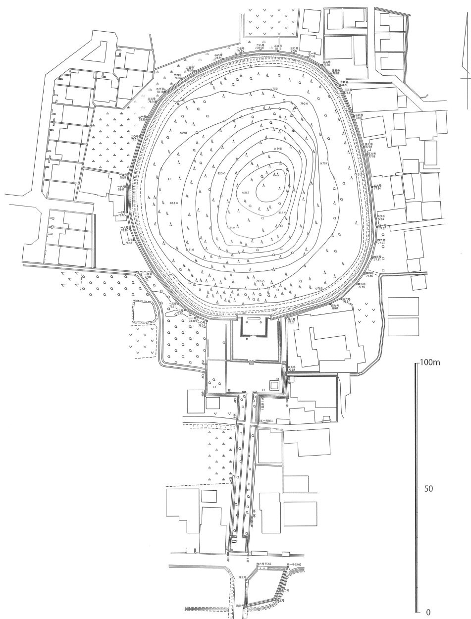
第49図 楊梅陵 測量図(1/1500)
