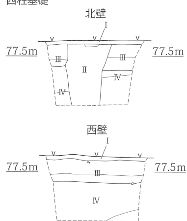
第51図 楊梅陵 掘削箇所断面図(1/80)
